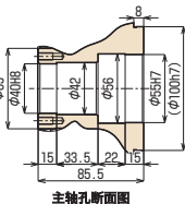
主轴承断面图
