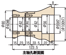
主轴承断面图
